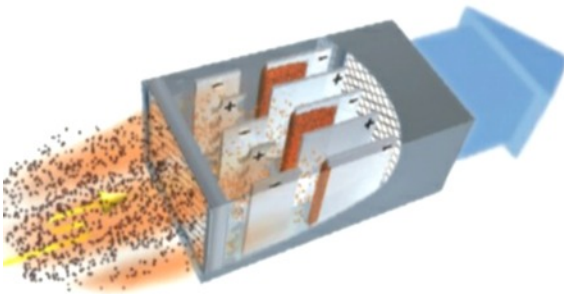
Funktionsweise Elektrofilter
